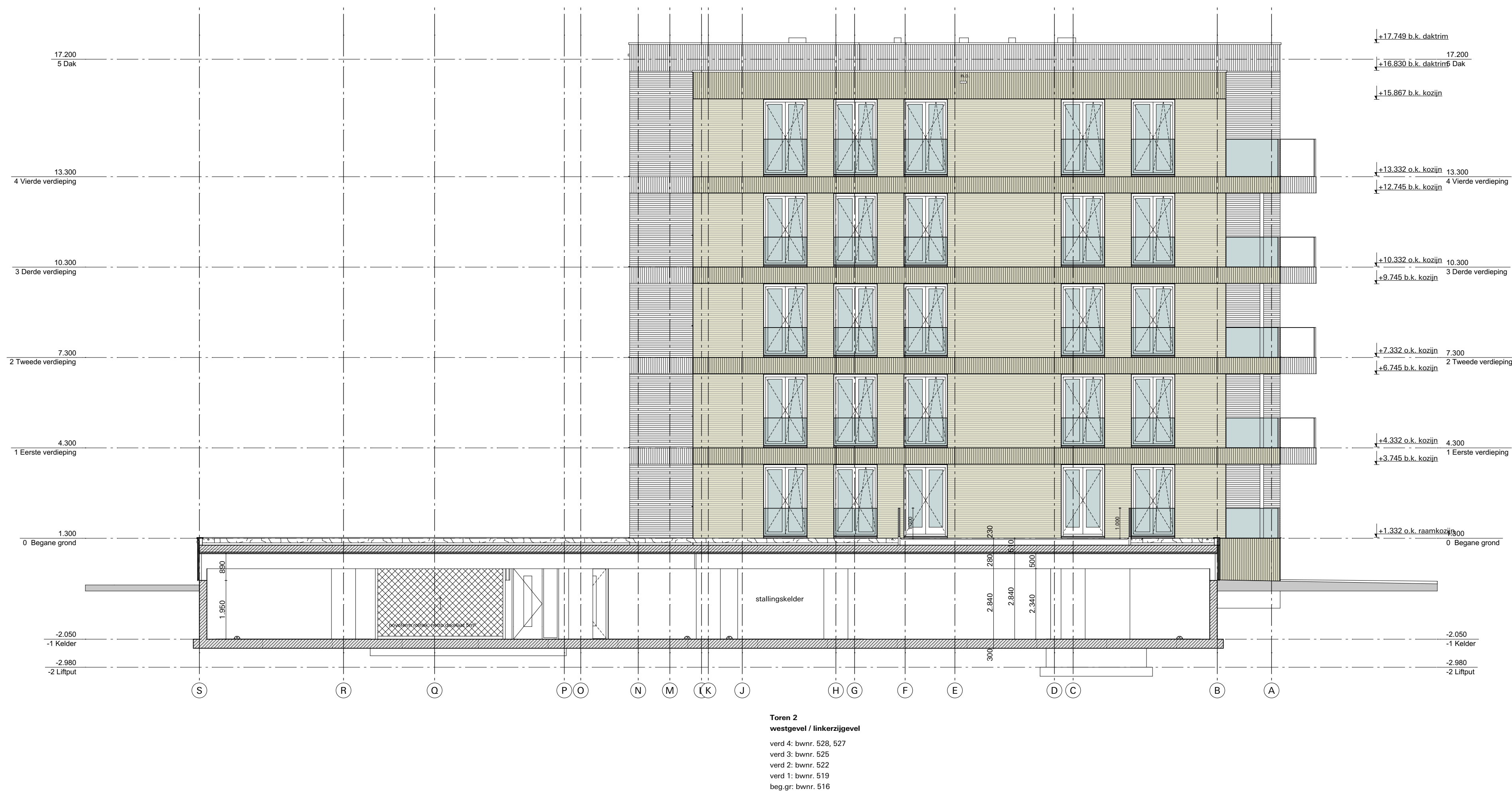
Doorsnede B-B schaal 1:100
