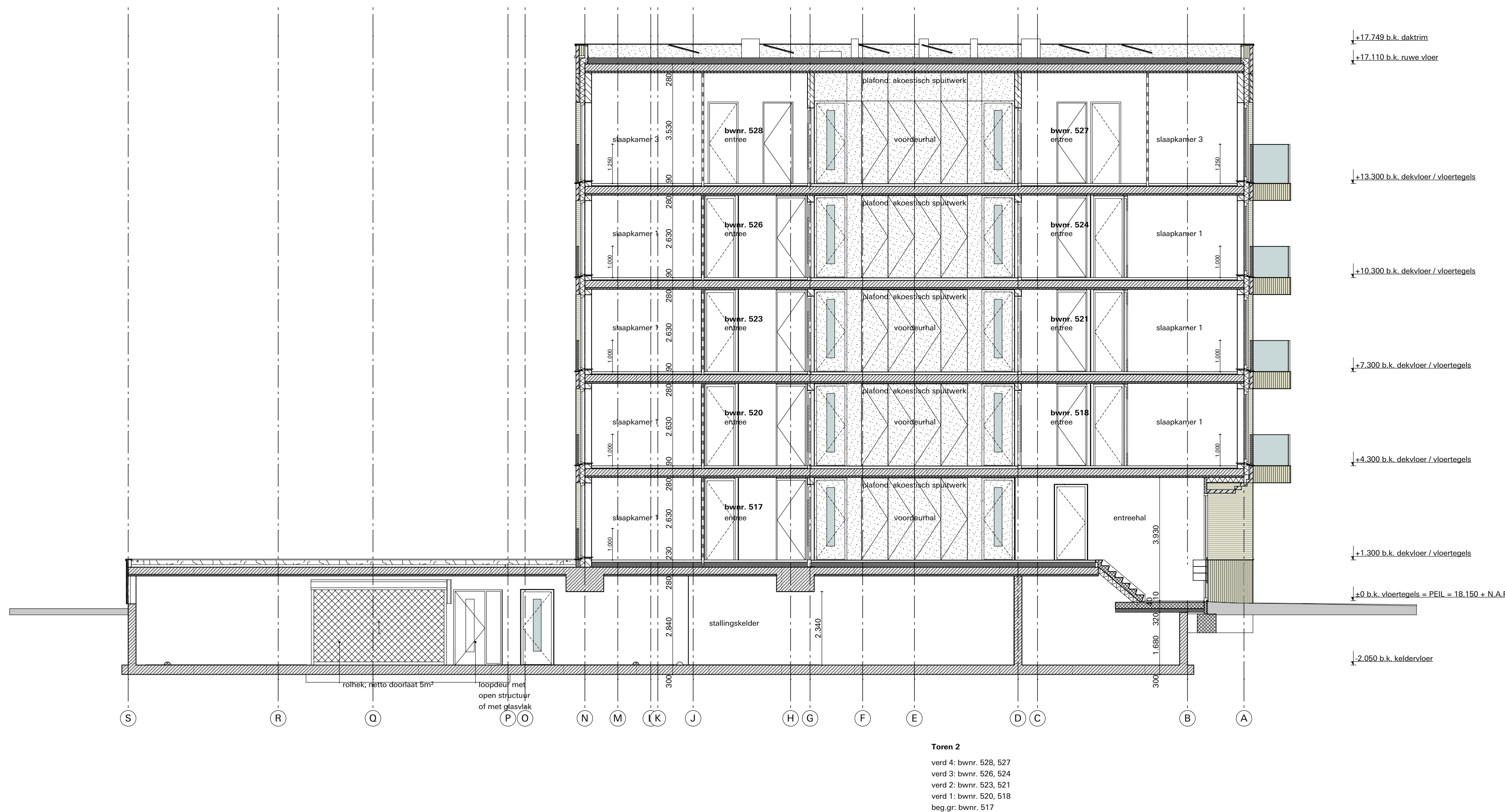
Doorsnede C-C schaal:100
